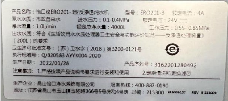
ERO201-3（铭牌）
